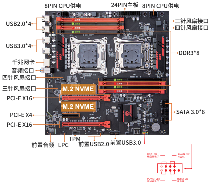
图1-1 X99-8D3双路主板图解
